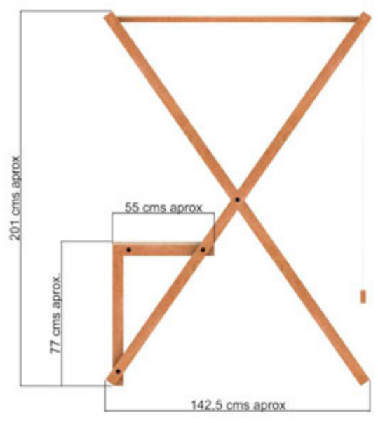
VISTA LATERAL
